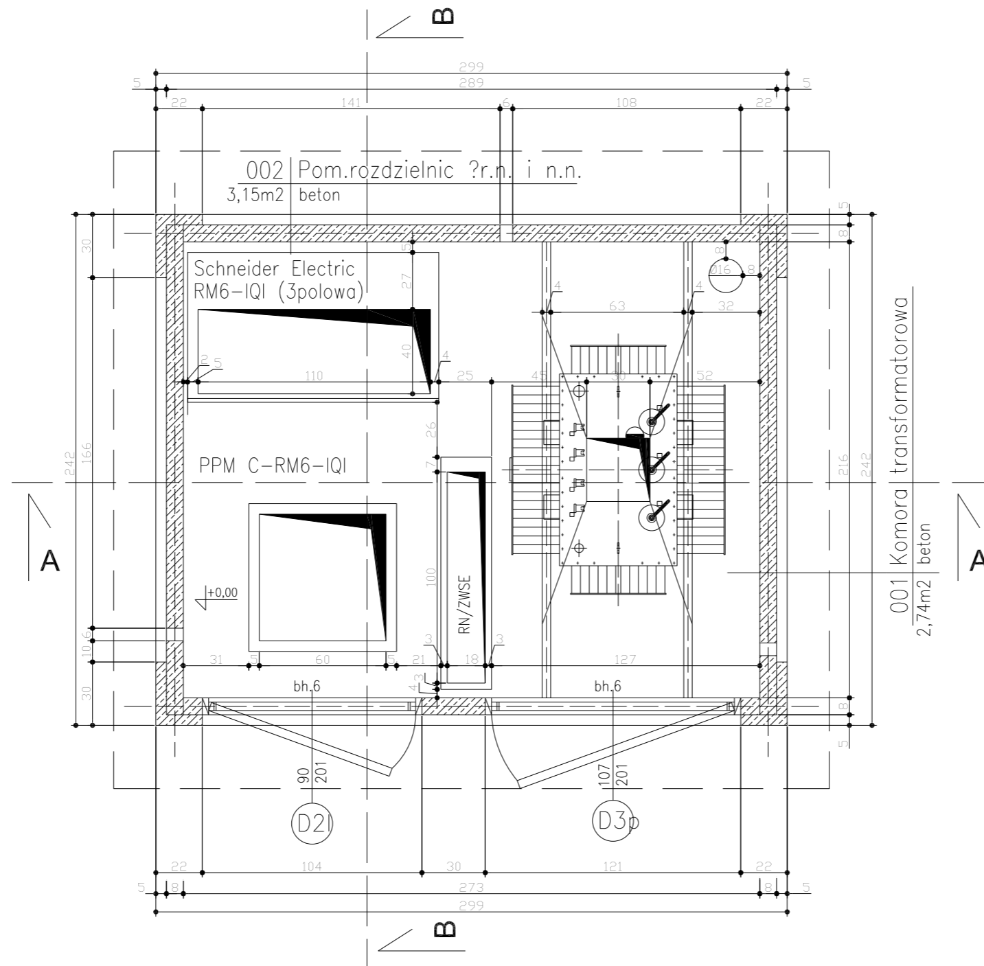
RZUT PRZYZIEMIA 1:25
