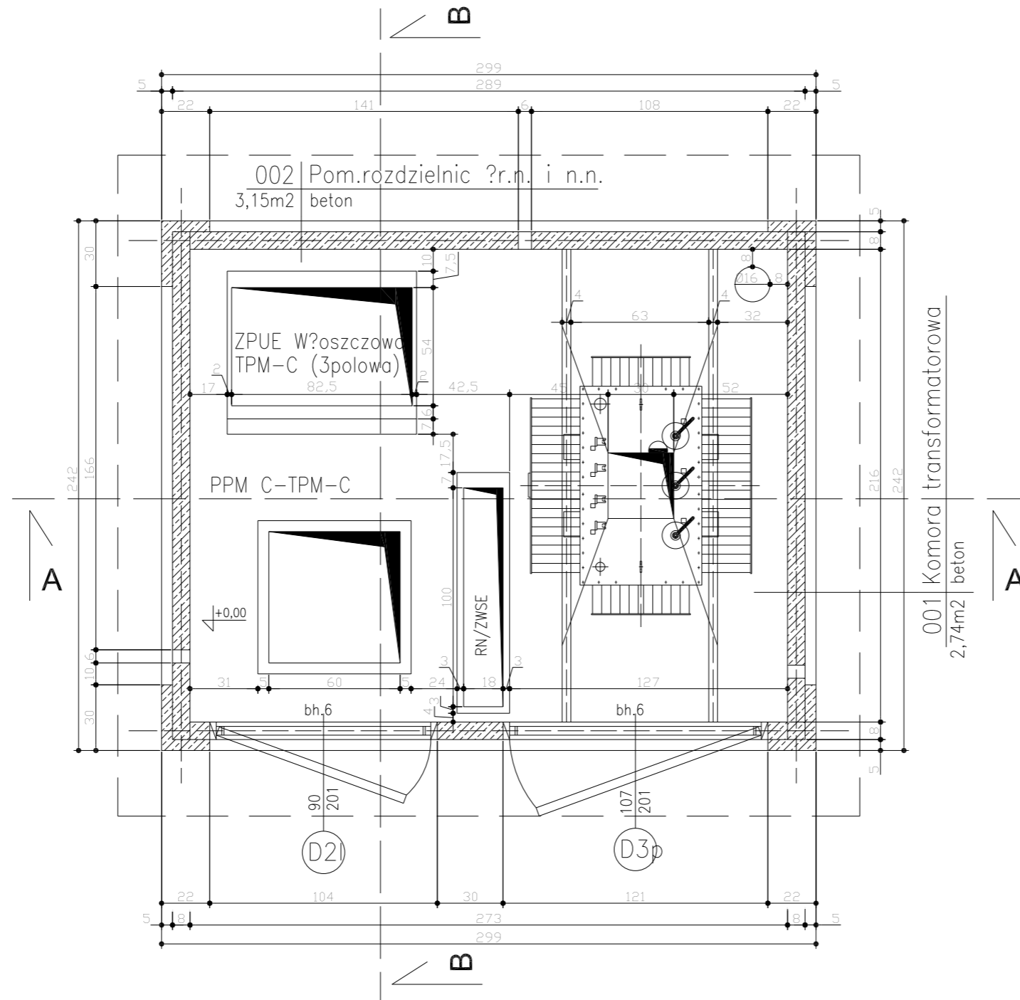
RZUT PRZYZIEMIA 1:25
