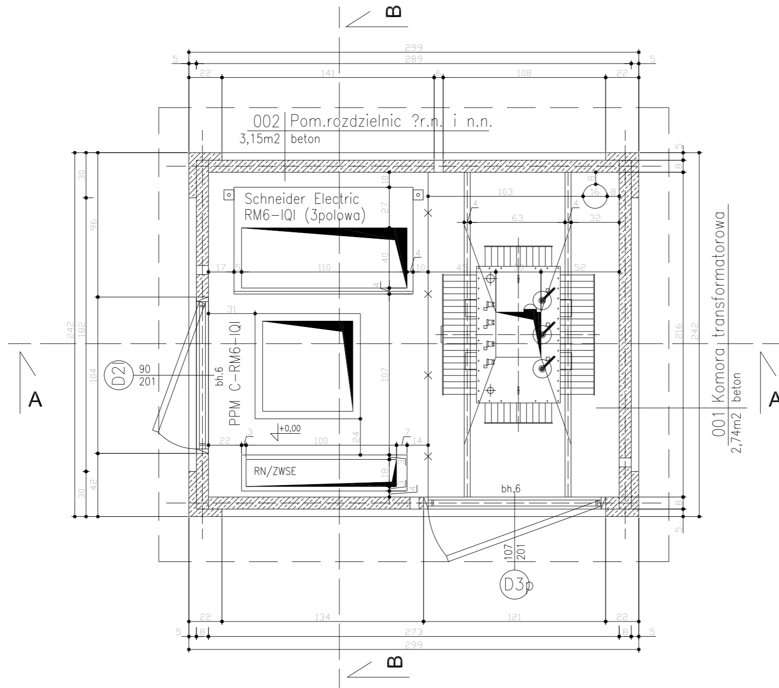
RZUT PRZYZIEMIA 1:25
