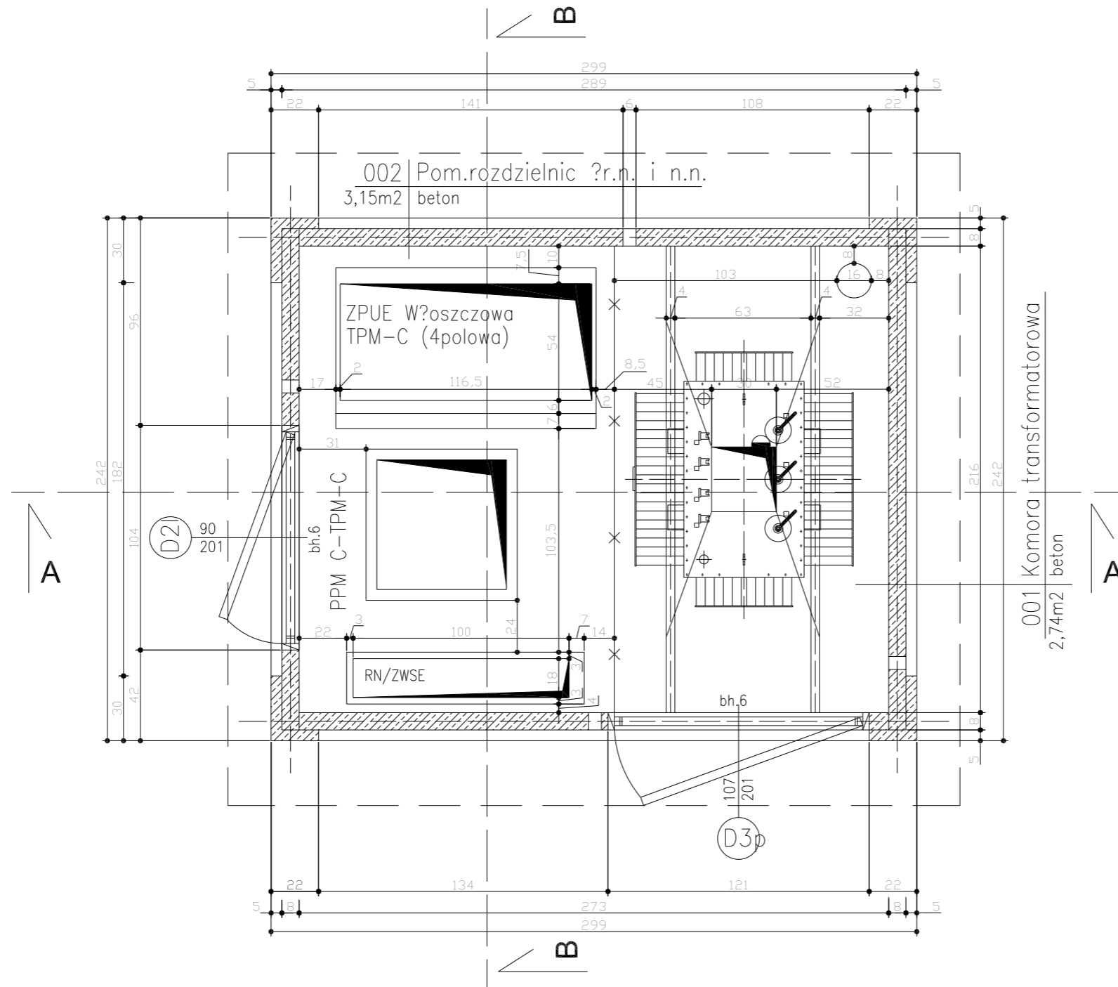
RZUT PRZYZIEMIA 1:25
