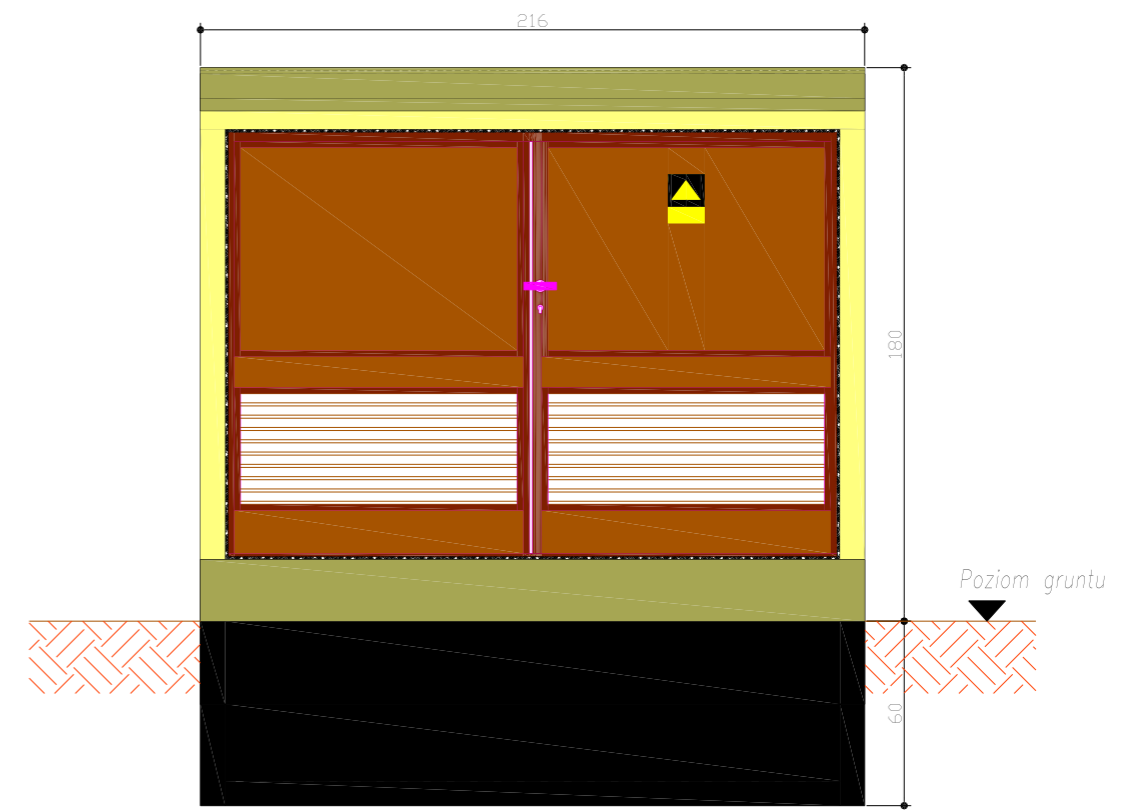
Elewacja frontowa 1:25 Elewacja tylna 1:25
