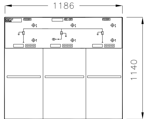
Rozdzielnica RM6 3-polowa
