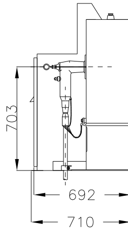
Rozdzielnica RM6 3-polowa
