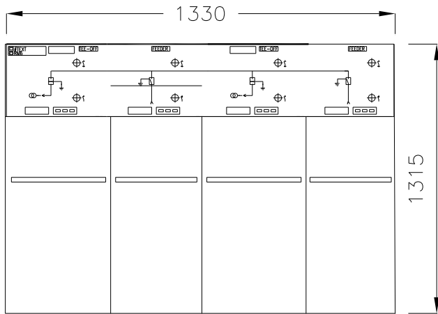
Rozdzielnica ALSTOM FBA 4001
