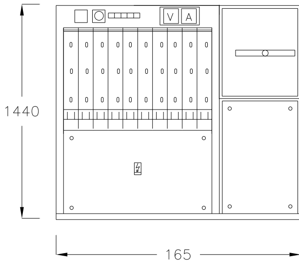
Rozdzielnice listwowe prod. Efen i Jane Mueller
