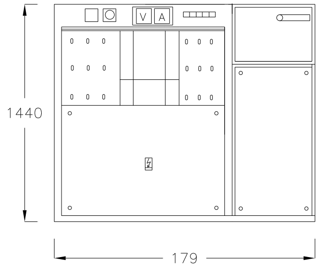
Rozdzielnice izolacyjne prod. ABB-Fastline
